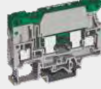
SFR.6/GR (6mm 2 sigortalı klemens)
